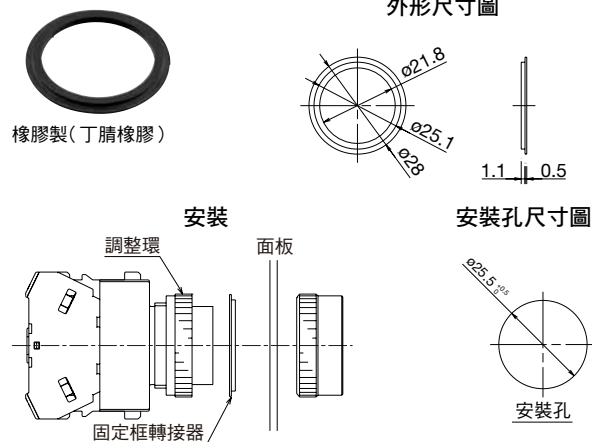
外形尺寸圖
