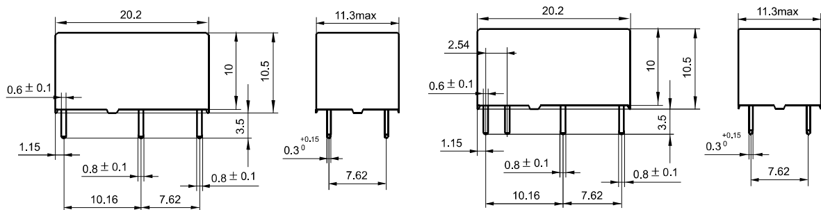
单稳态、单线圈磁保持
