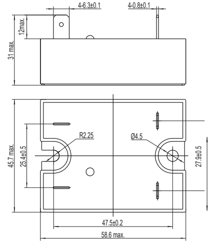
(016) 安装尺寸图
