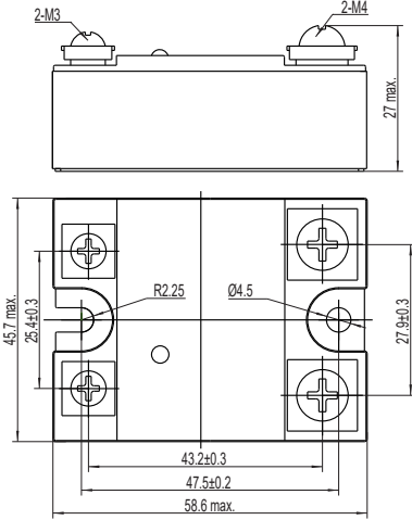
常规安装尺寸图
